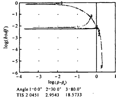
图1 Aeroglaze 漆的多项式模型
