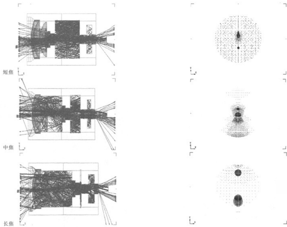
图3 变焦系统的鬼像模拟和点列图
