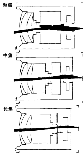
图 7 路径的光线追迹
