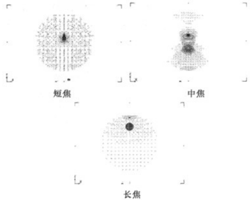
图 6 优化后的点列图
