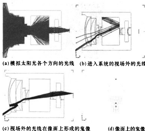
图10 视场外的光线在系统形成的鬼像
