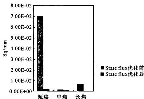
图9 优化前后能量比较
